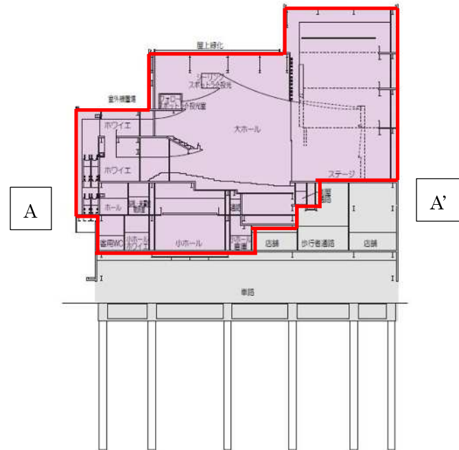
(大ホール等断面図)
