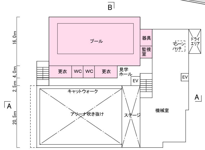
地下1階平面計画図
