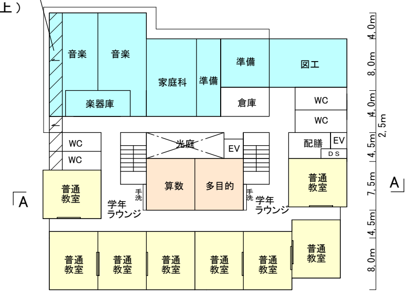
3階平面計画図
