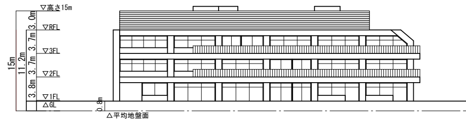
北側立面
