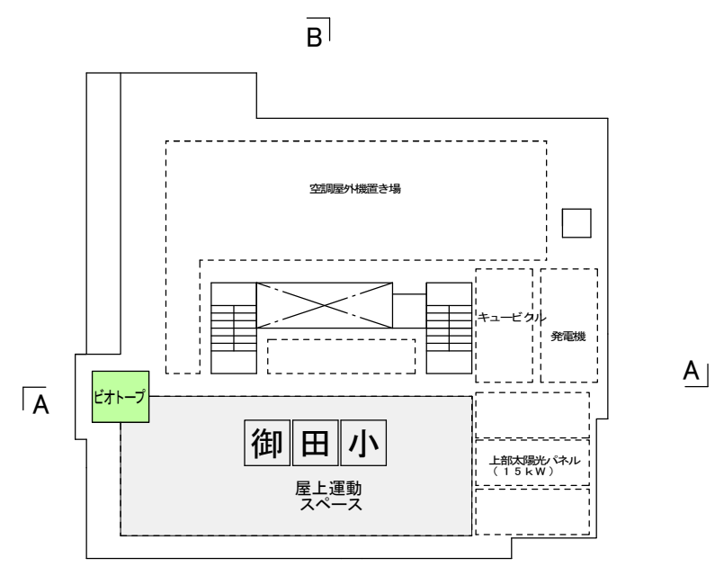
屋上平面計画図
