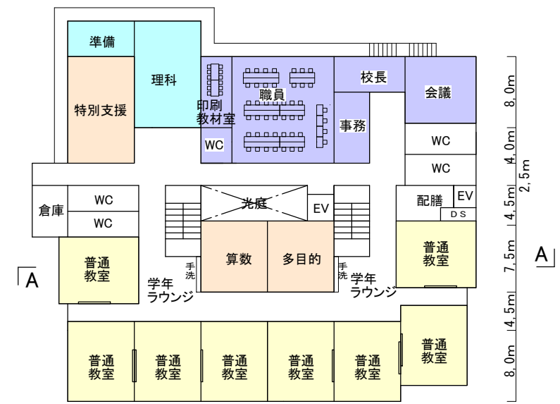
2階平面計画図
