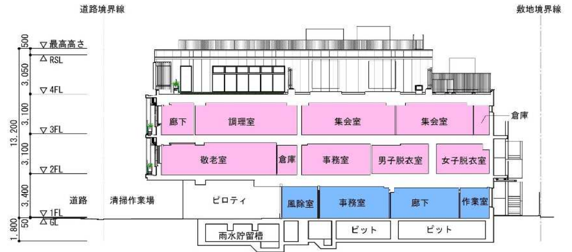
B-B' 断面図
