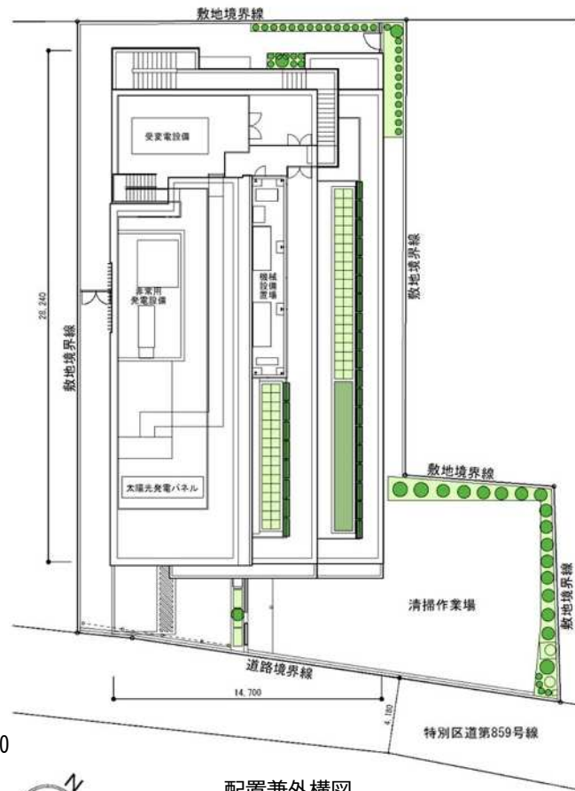
配置兼外構図
