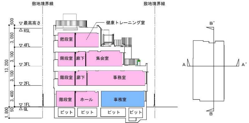
A-A' 断面図
