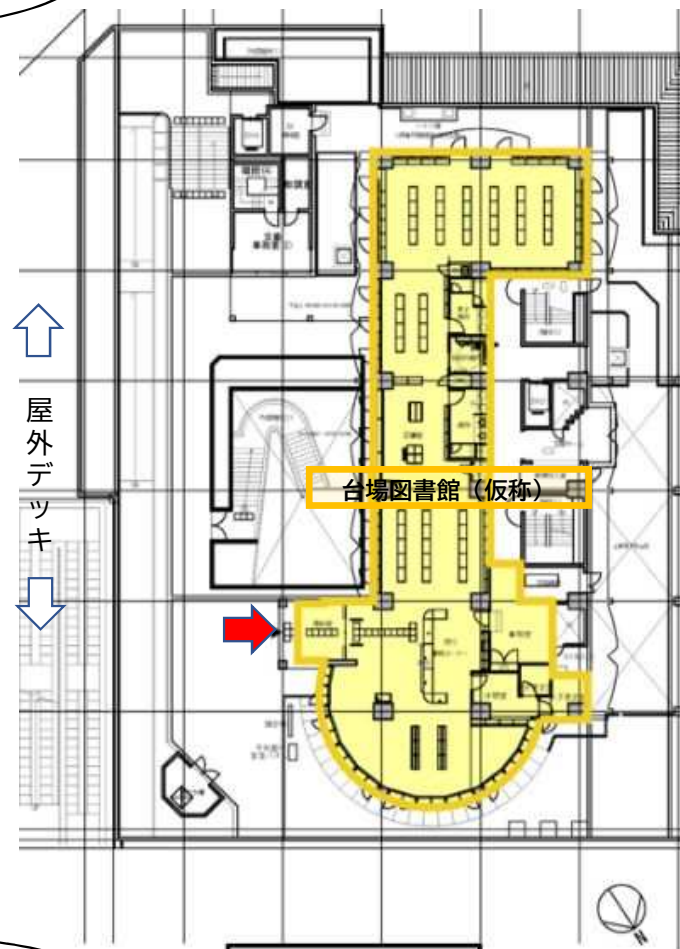
3階平面図
