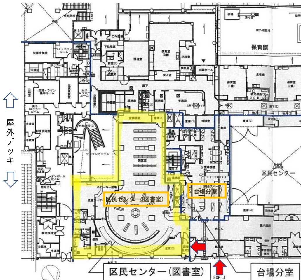
2階平面図
