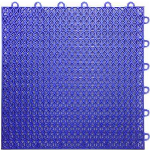
W300mm×H300mm×D15mm
