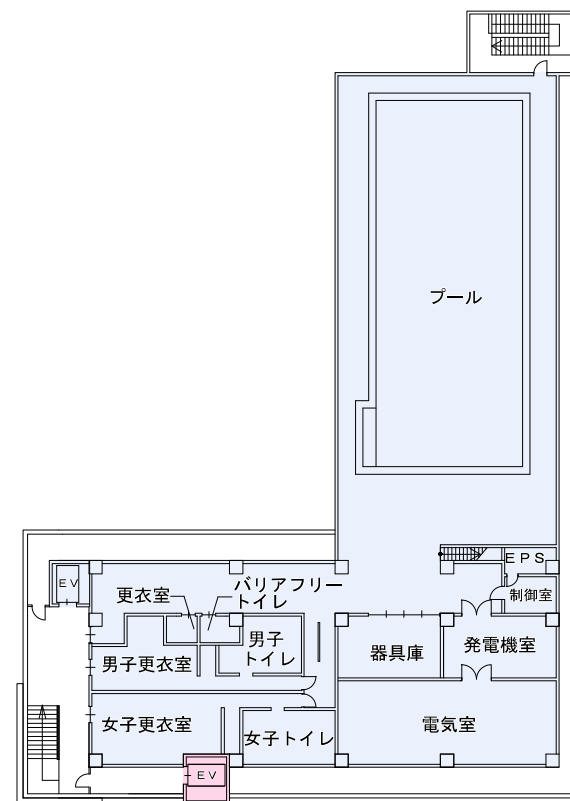
5階
