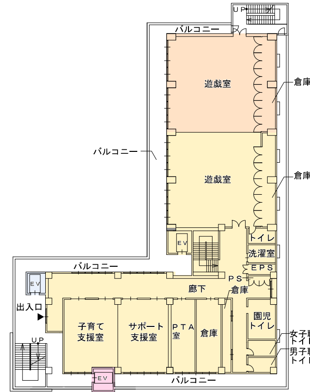
2階
