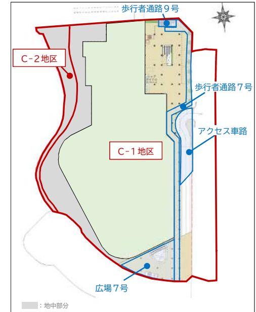
■配置図(案)：1階（地上レベル）
