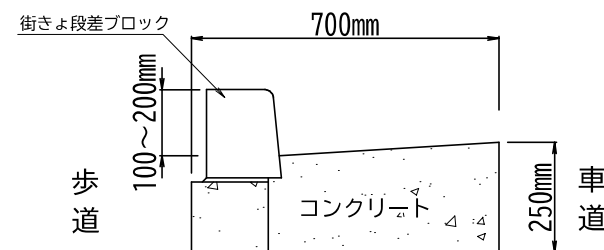
街きよ断面図(変更後)
