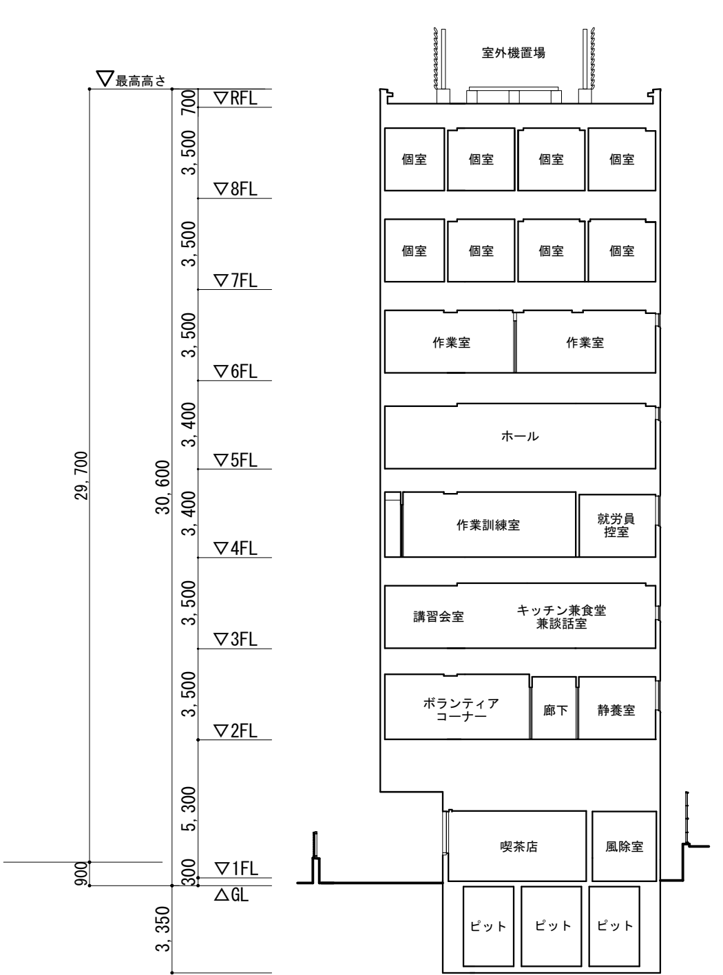
B-B' 断面図
