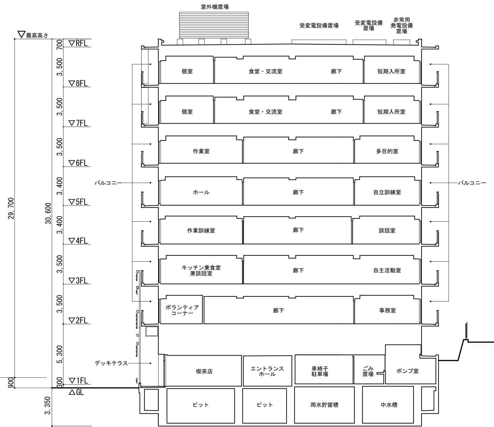
A-A' 断面図
