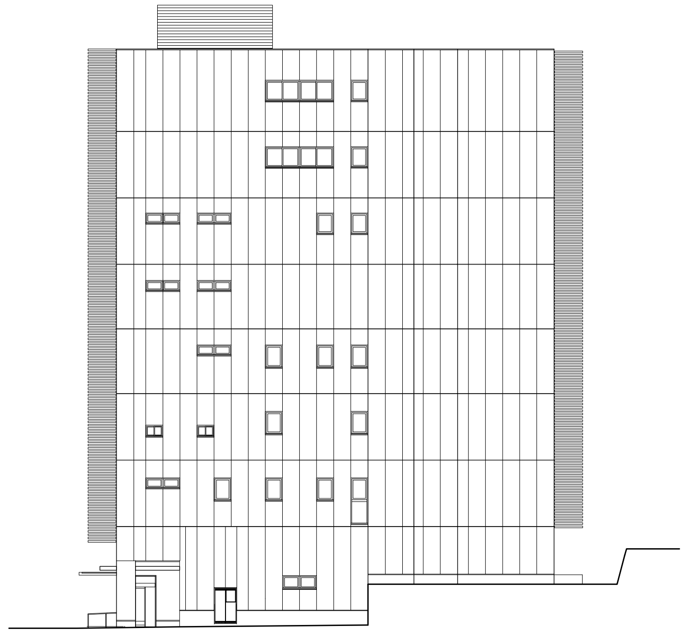
西側立面図
