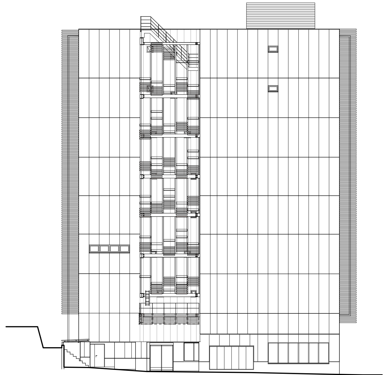
東側立面図
