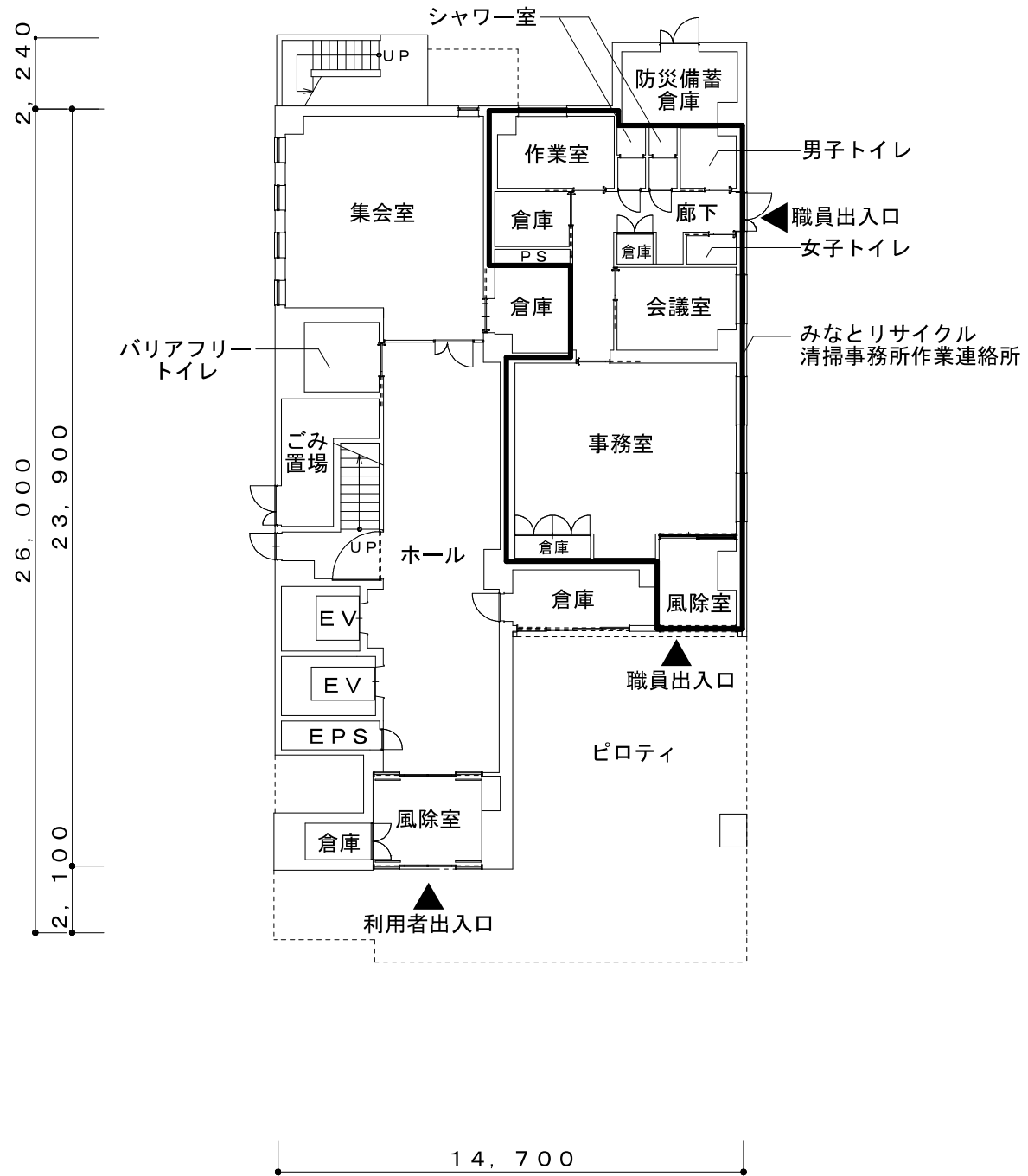
1階平面図
