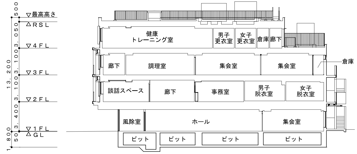
B—B' 断面図
