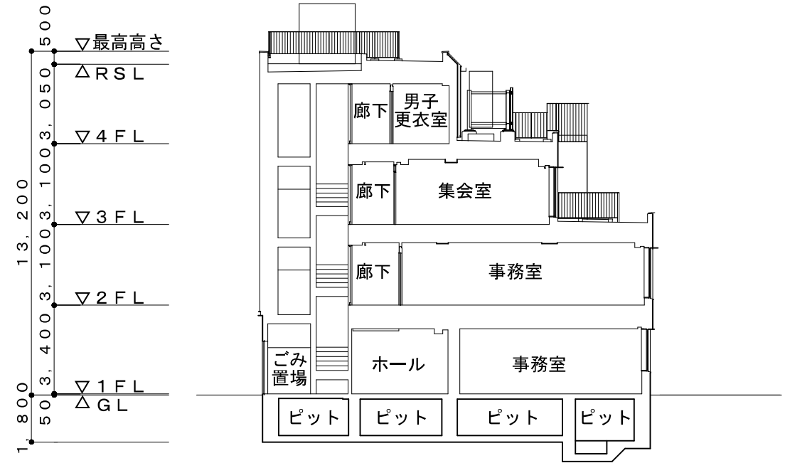
A—A' 断面図
