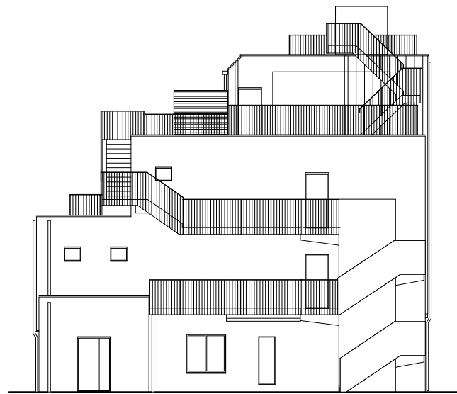
北側立面図
