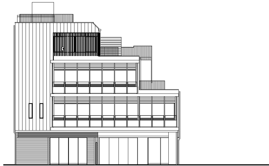
南側立面図
