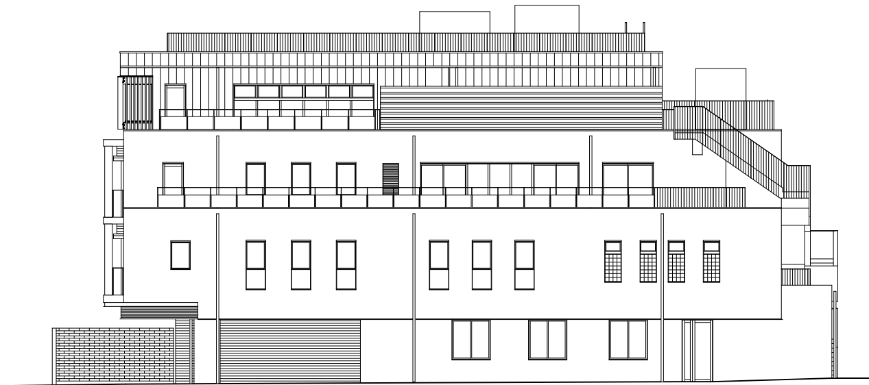
東側立面図
