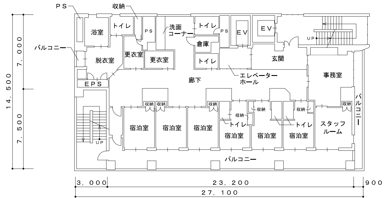
3階平面図
