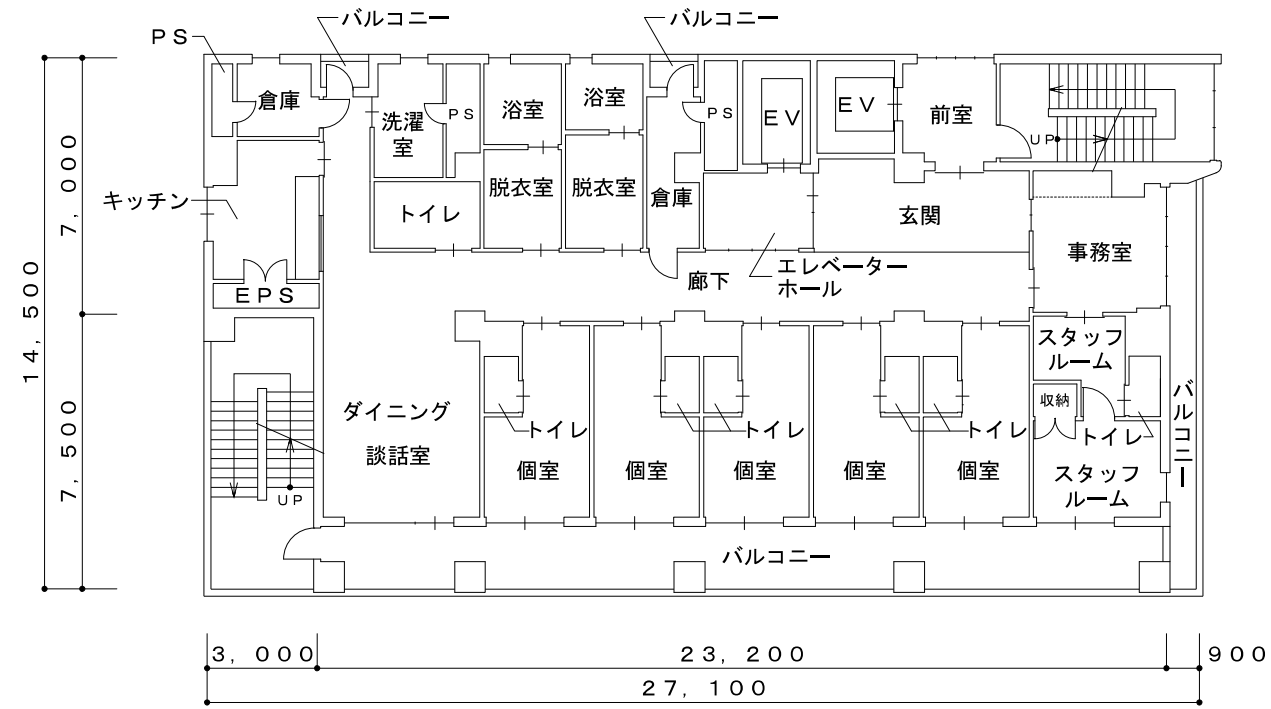
4階平面図
