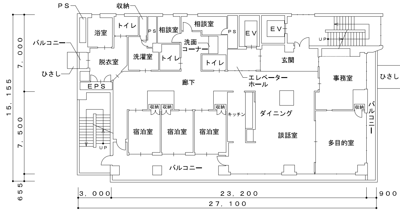
2階平面図
