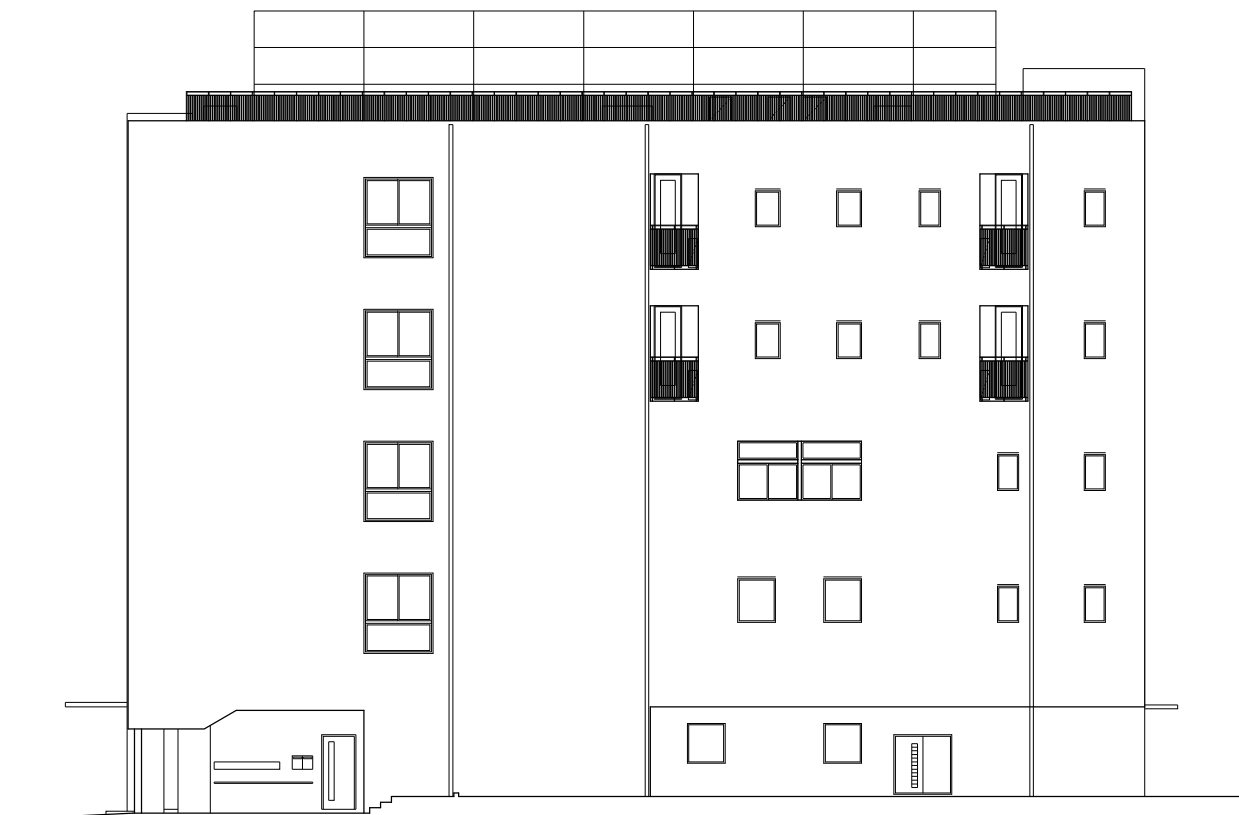
北側立面図
