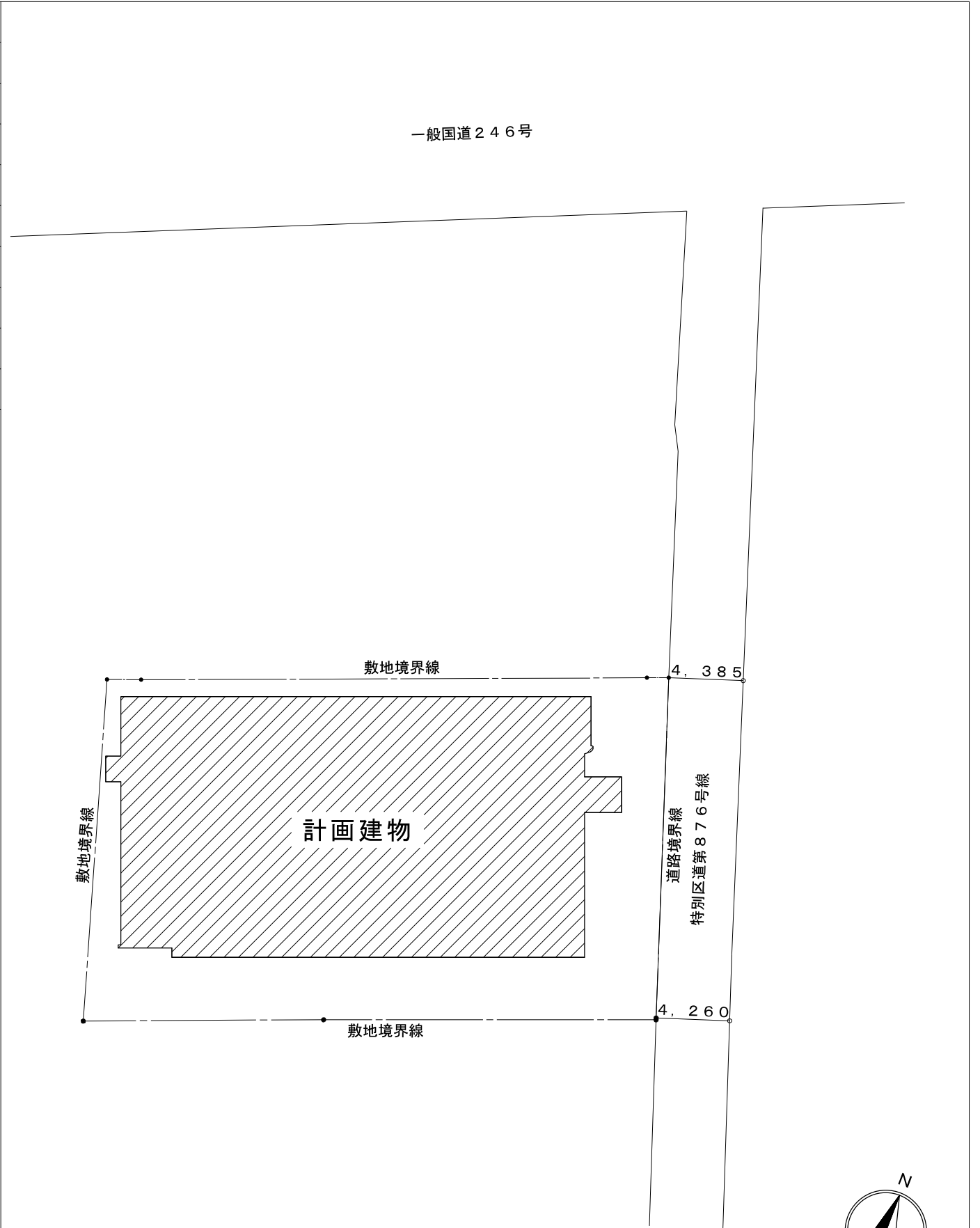
配置図 縮尺 1 / 300
