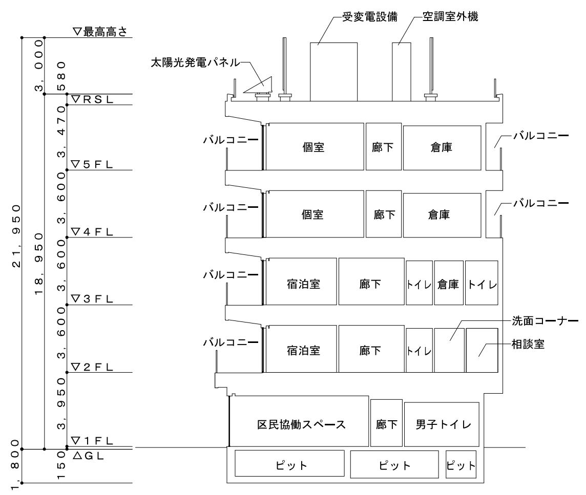
A-A' 断面図
