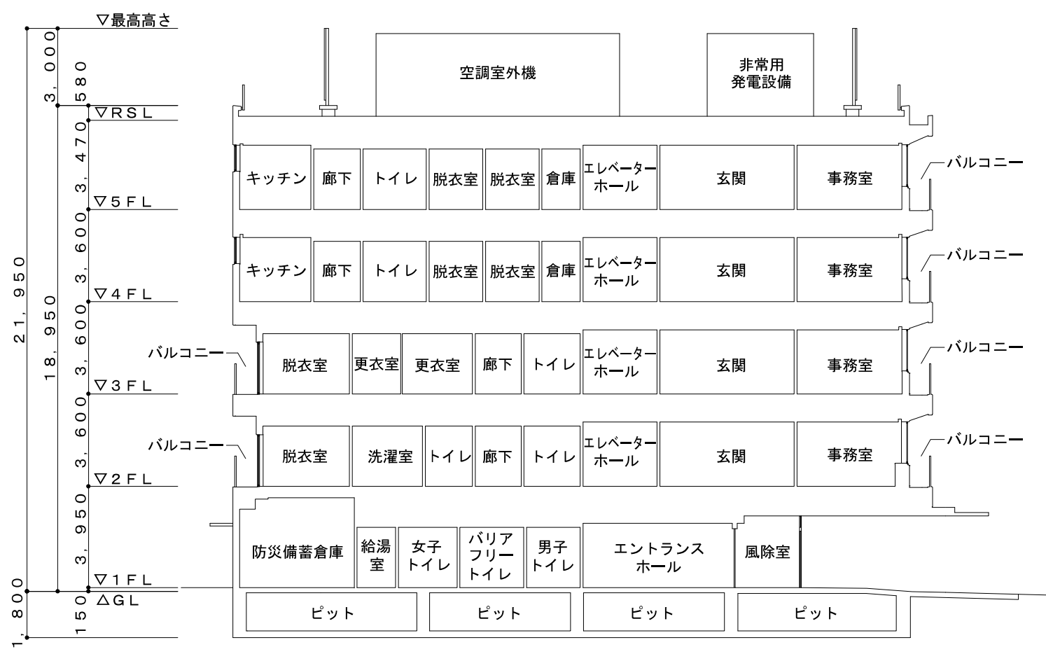
B-B' 断面図
