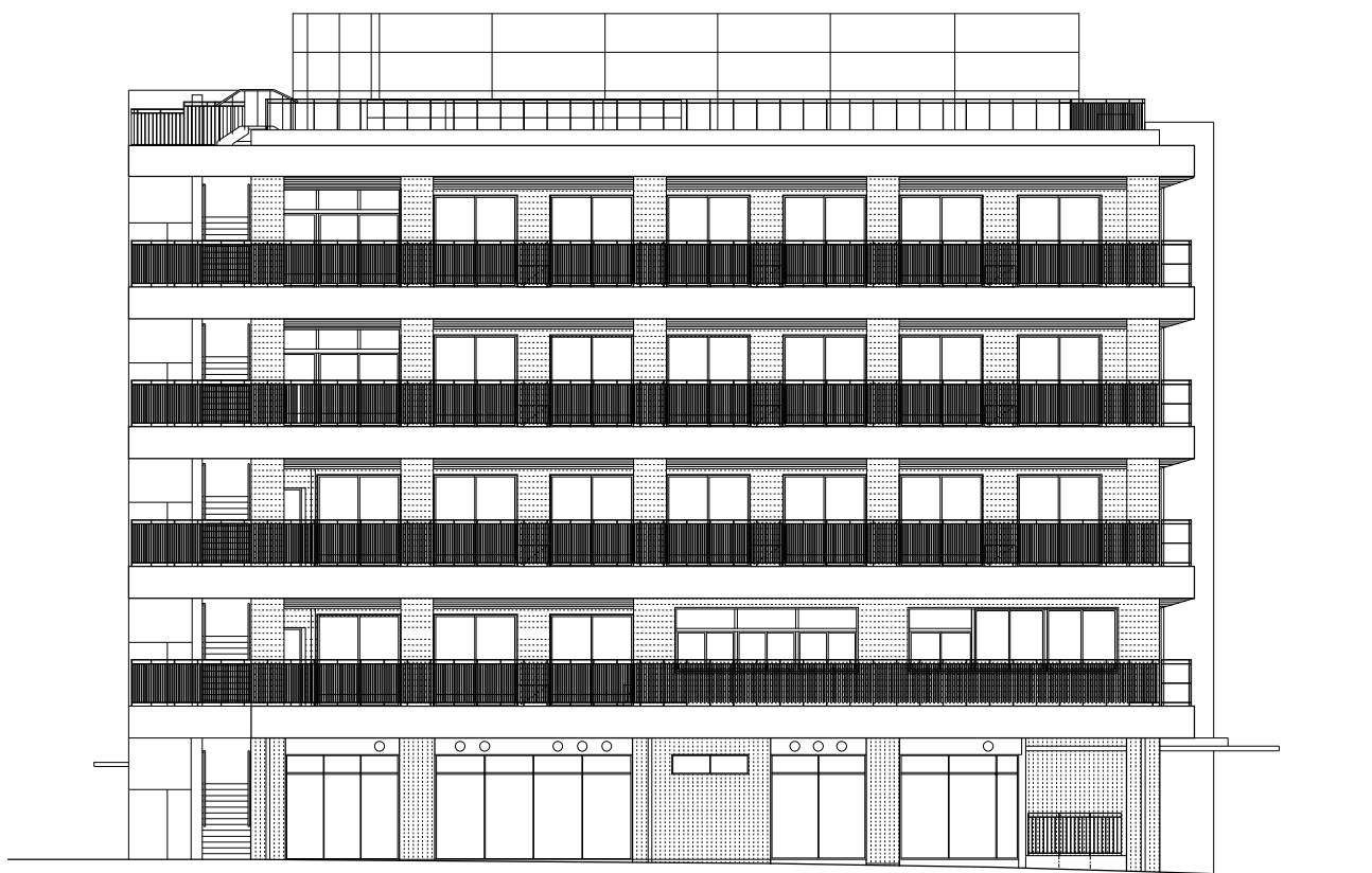
南側立面図
