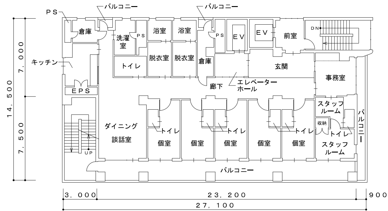
5階平面図
