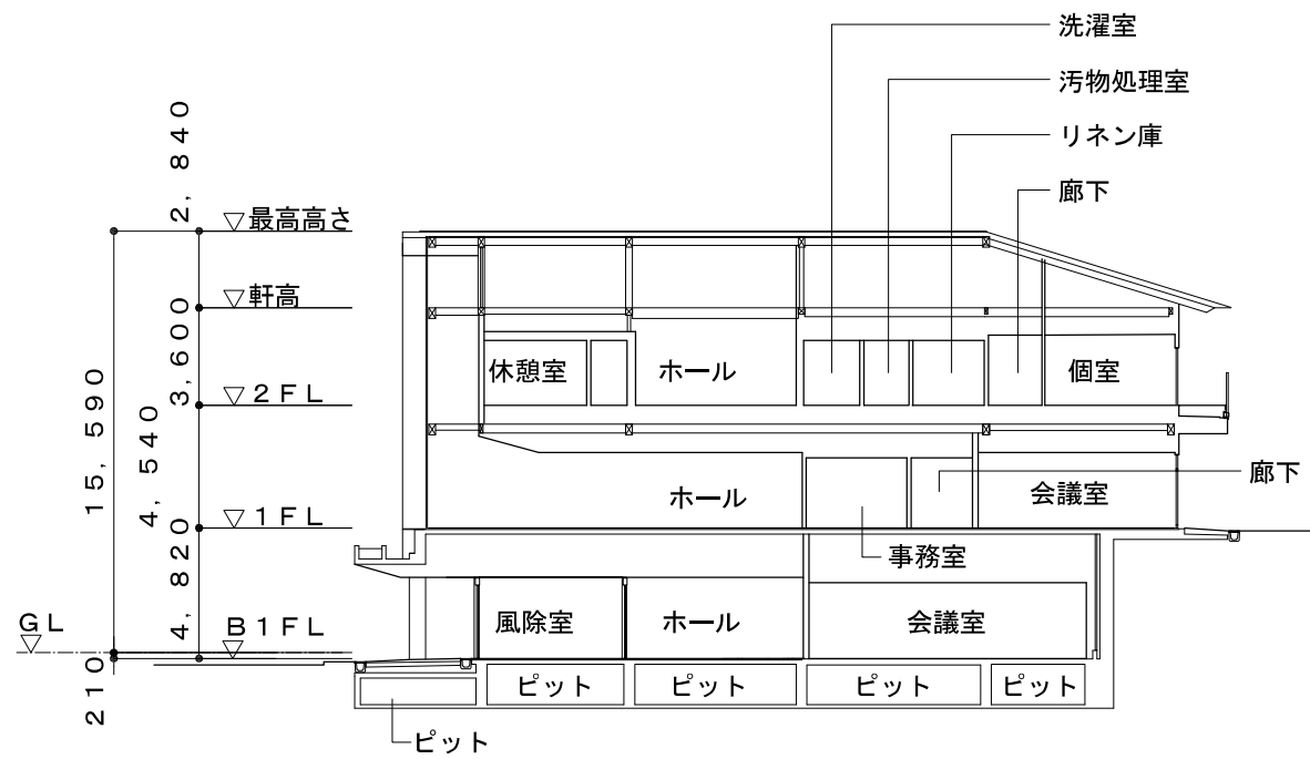
A-A' 断面図
