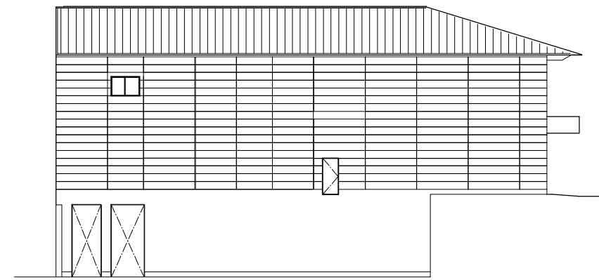
東側立面図
