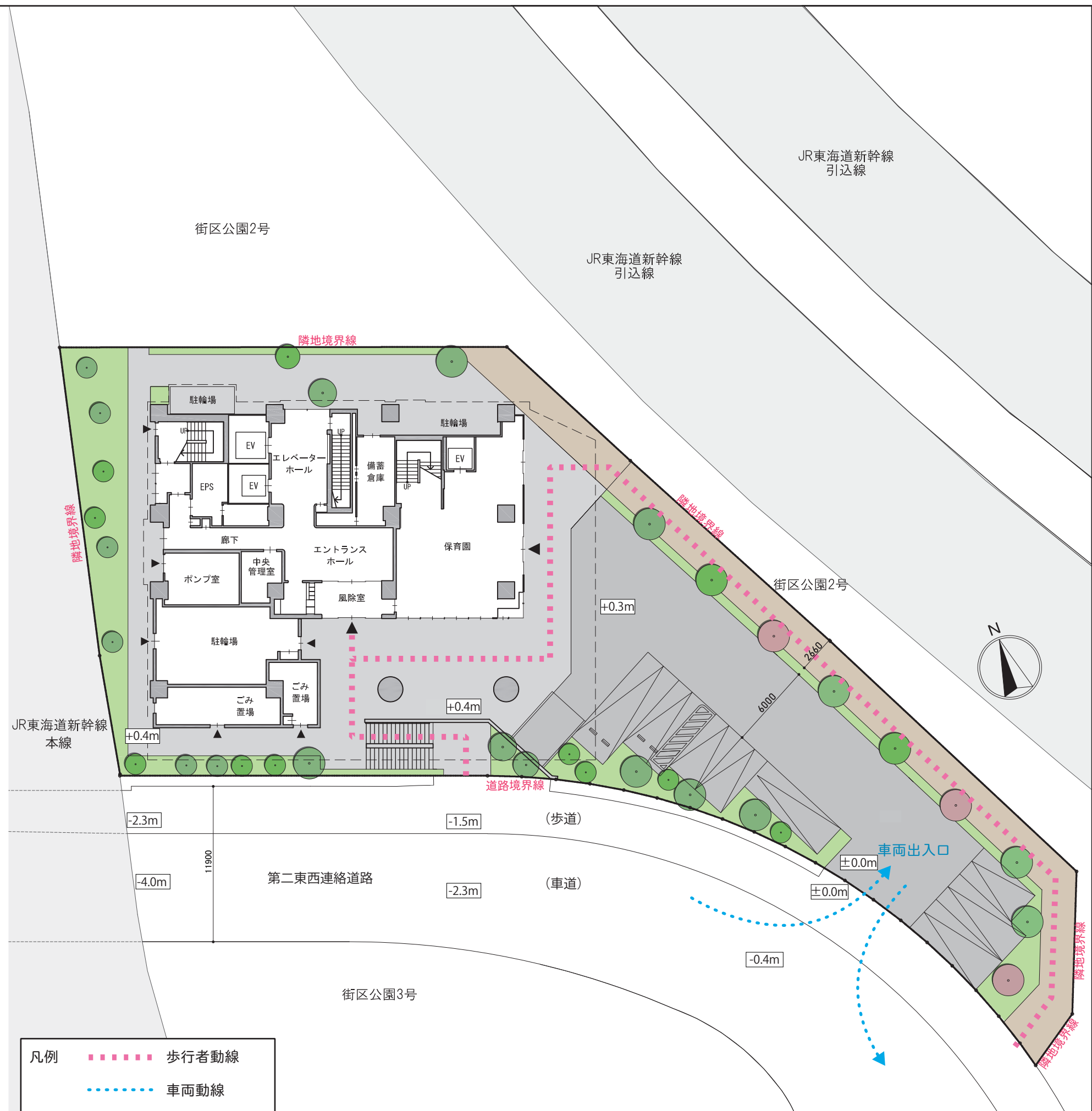
配置図兼一階平面図 No scale
