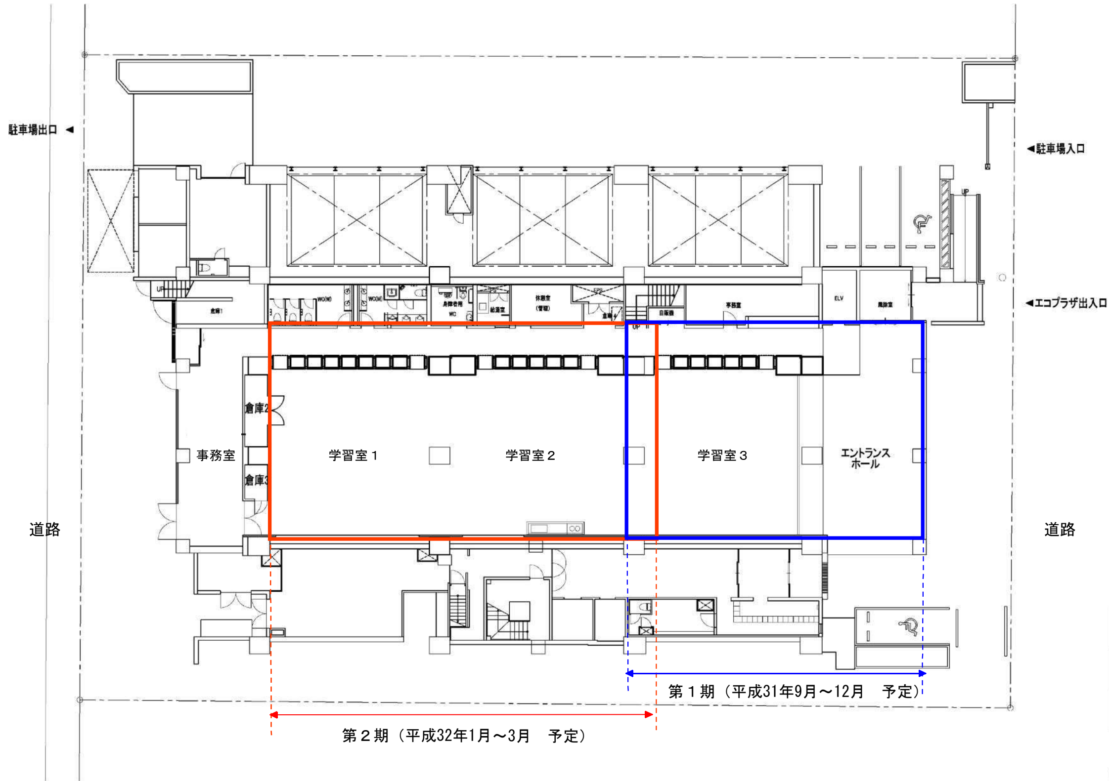
(1階平面図)
