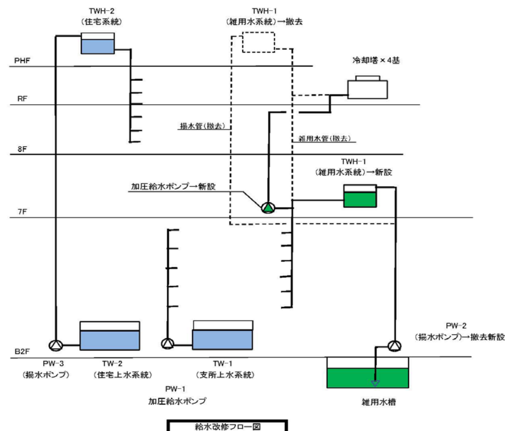
給水改修フロー図
