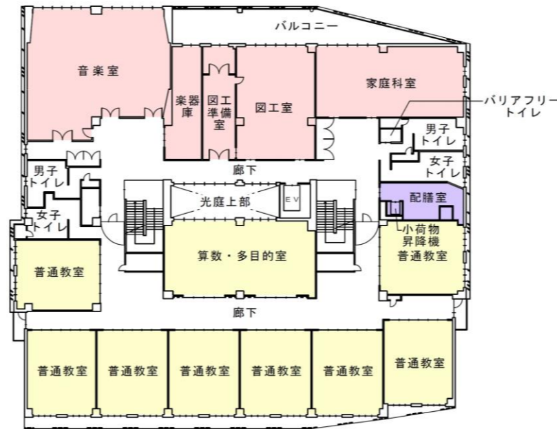
3階平面図
