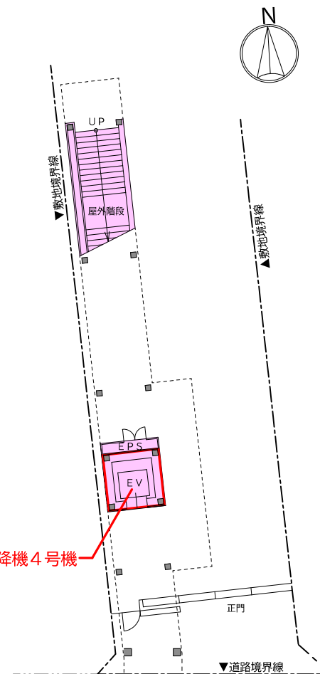
連絡通路 1階平面図 Scale:1/200
