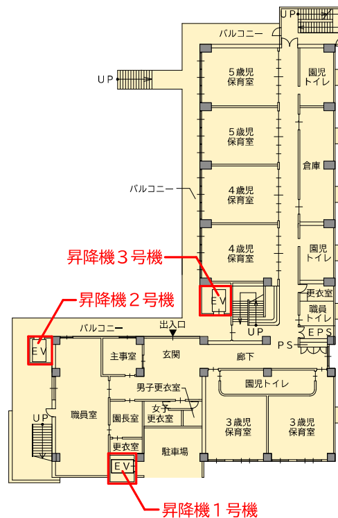
園舎等複合施設棟 1階平面図 Scale:1/500
