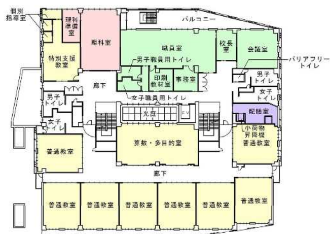
2階平面図
