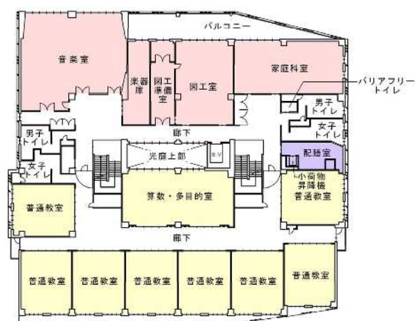
3階平面図
