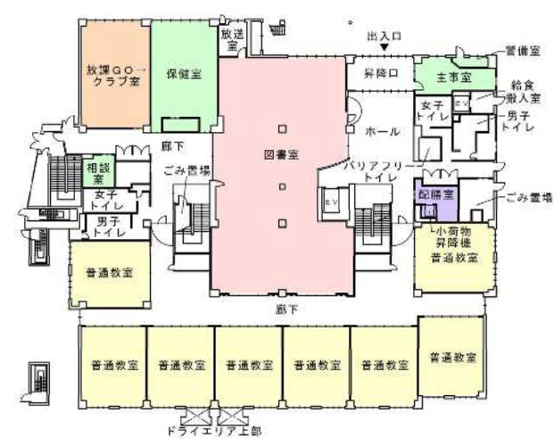
1階平面図
