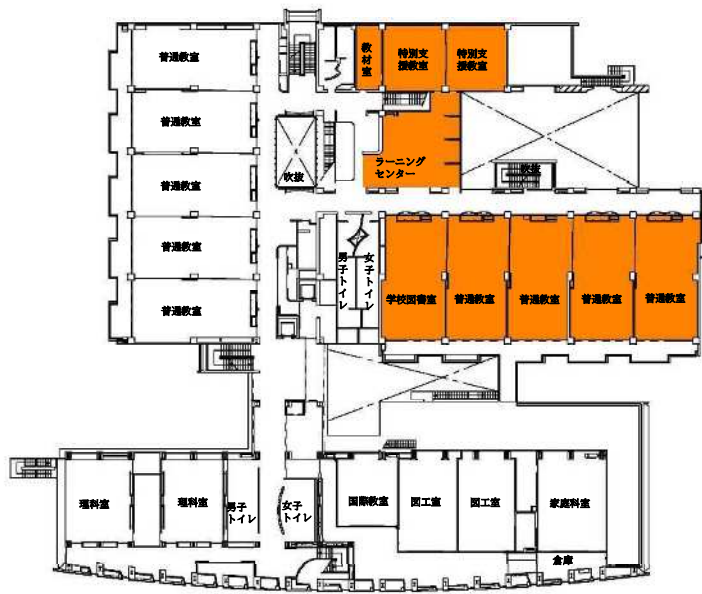
3階平面図
