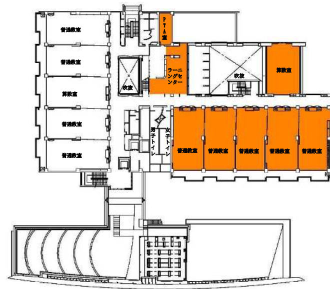
4階平面図
