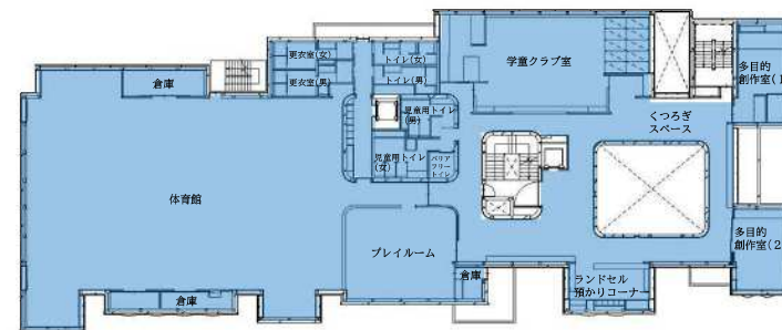
2 階平面図
