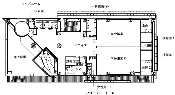
8階平面図
