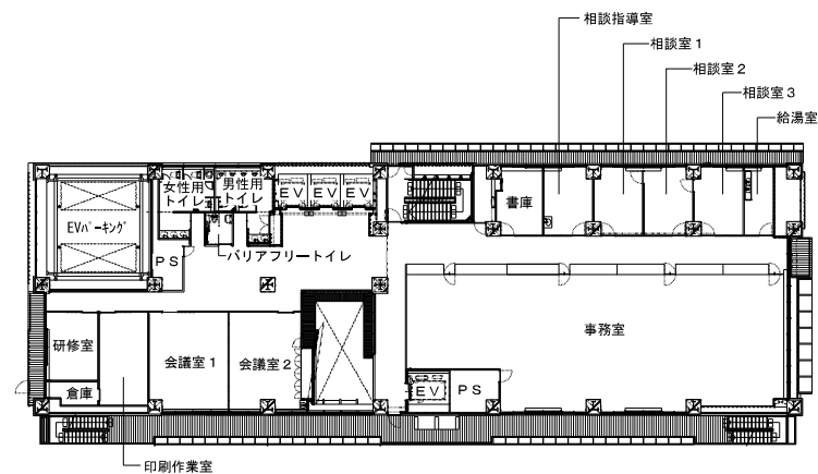
4階平面図
