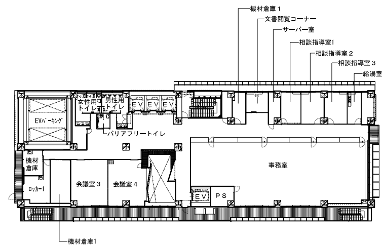
5階平面図
