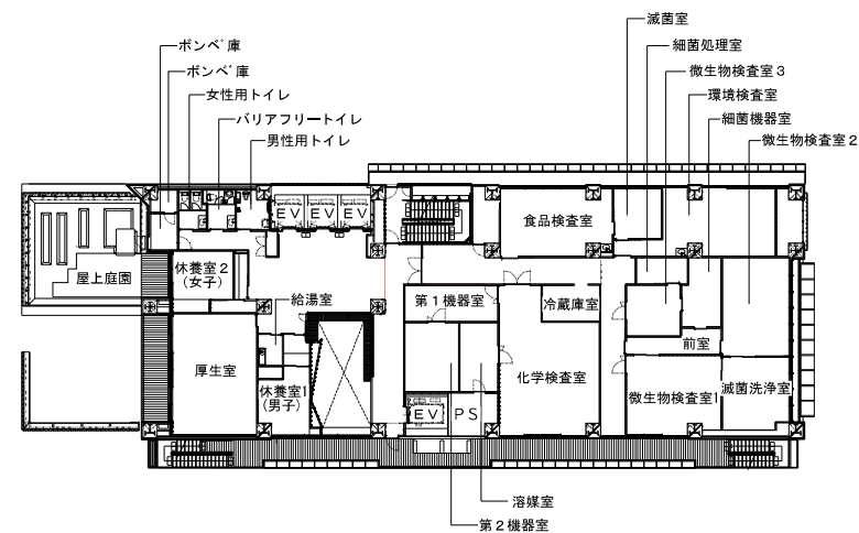
7階平面図
