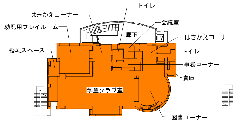
地下1階平面図
