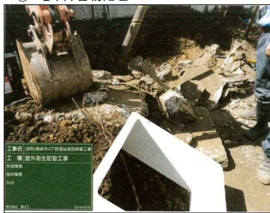
② 下水道接続工事に伴う試掘
