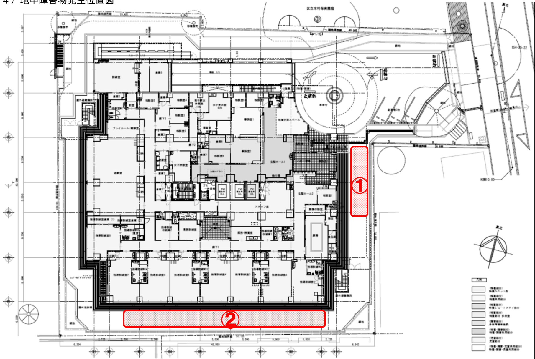
(4) 地中障害物発生位置図
